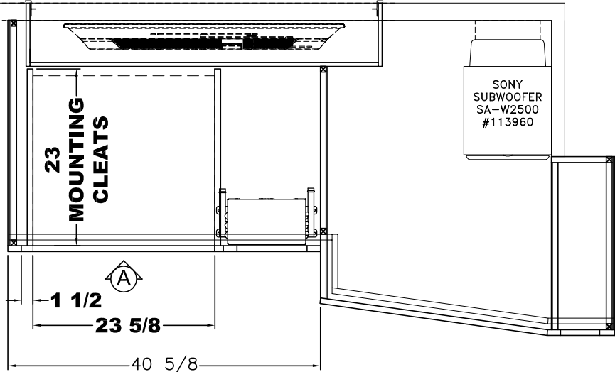
PLAN (J525)
