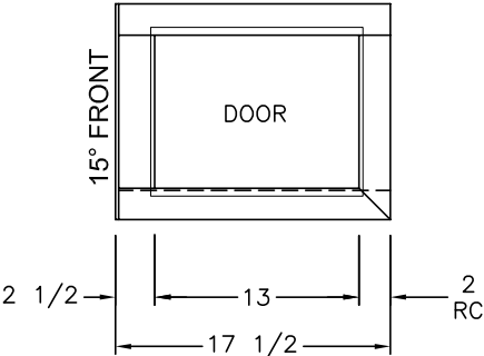
(1) 13 1/2 X 10 3/4 DOOR (TOP HINGE)
