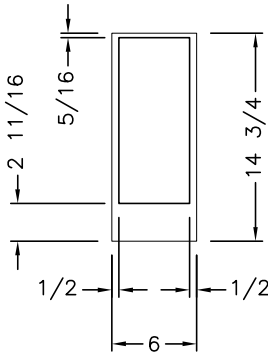
DOOR OVERLAY
