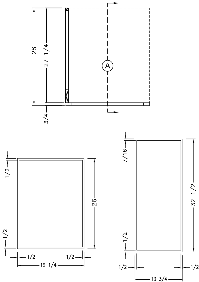
DOOR OVERLAYS
