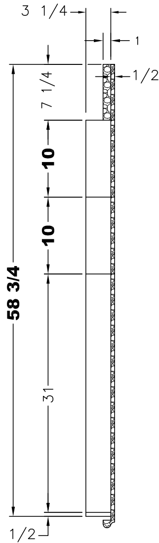
SECTION A-A
