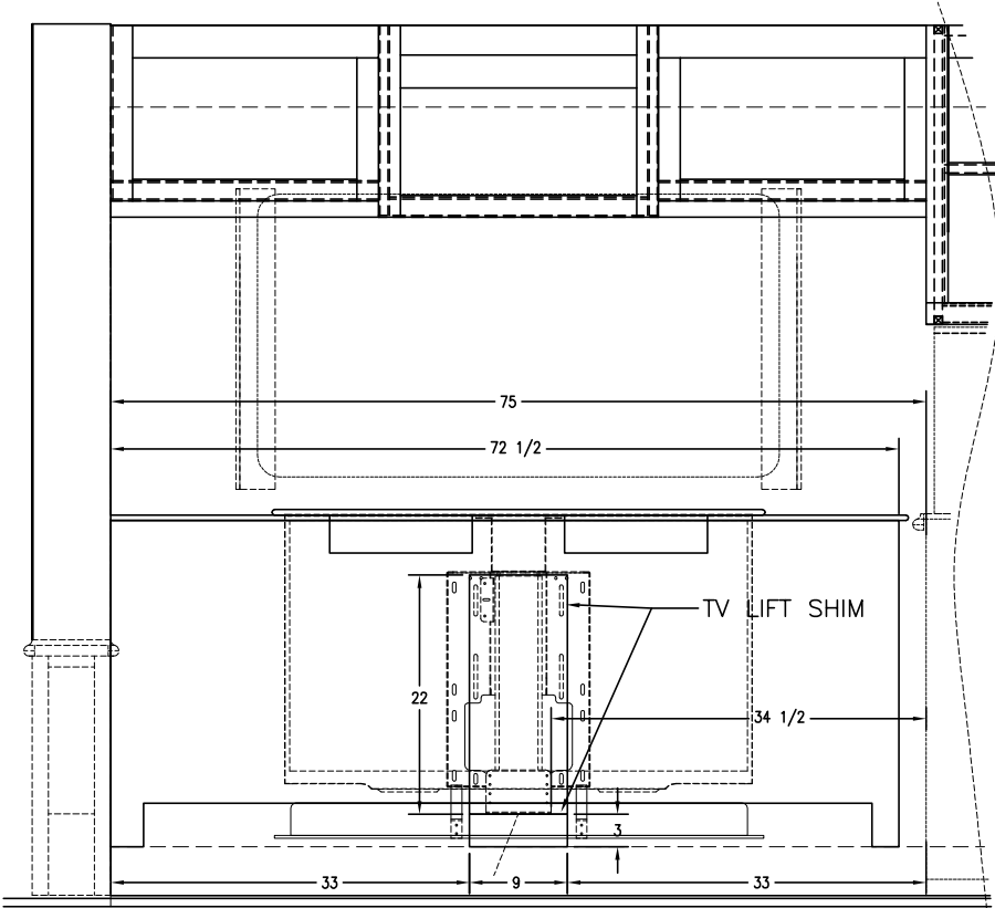
ELEVATION
