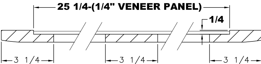
D-D (ENLARGED 5X)
