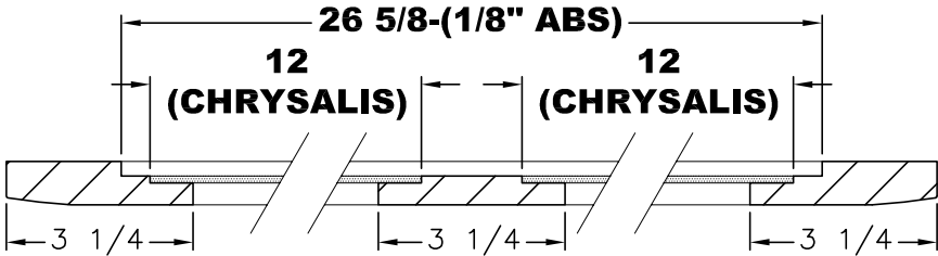
D-D
