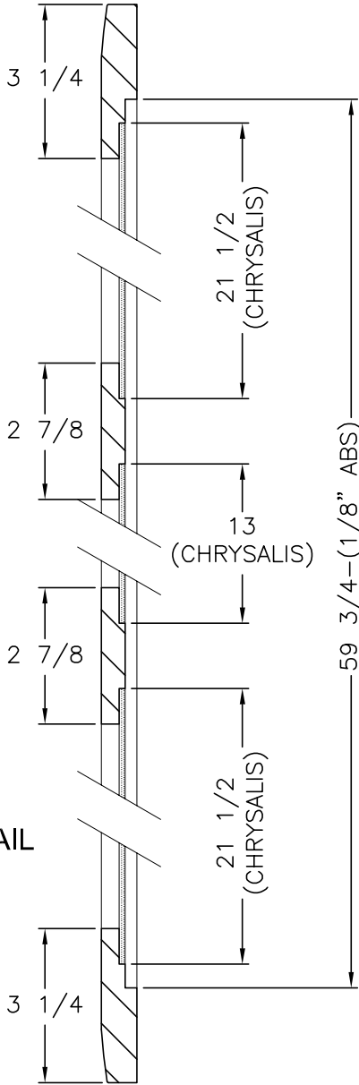
C-C
