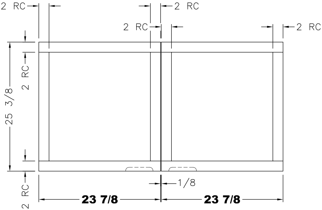
DOOR FRAMES
