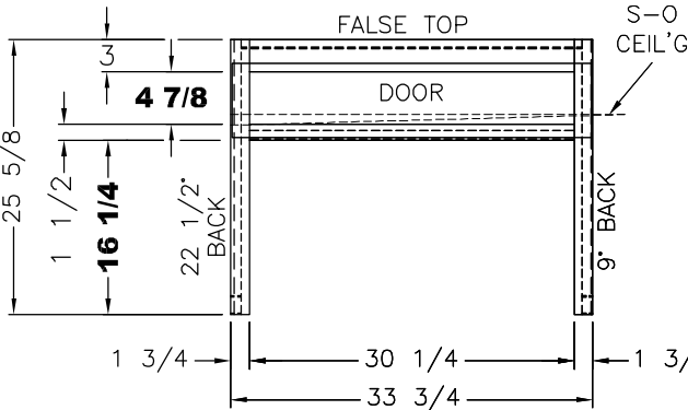
(1) 33 1/2 X 6 7/8 DOOR (TOP HG)
