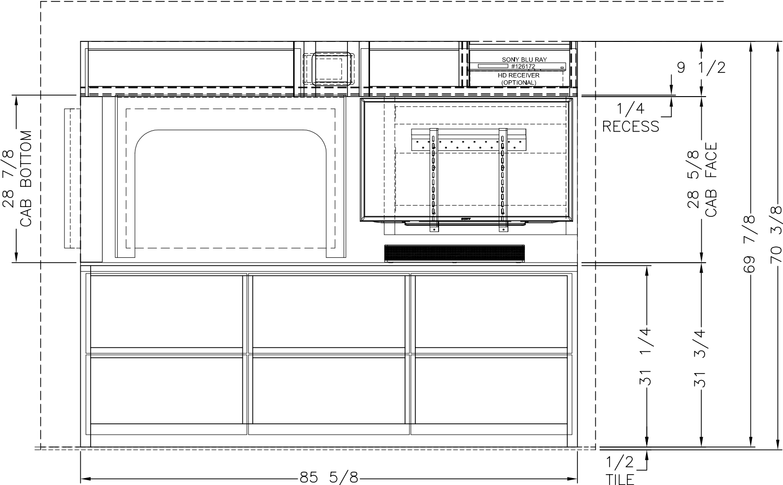
ELEVATION
