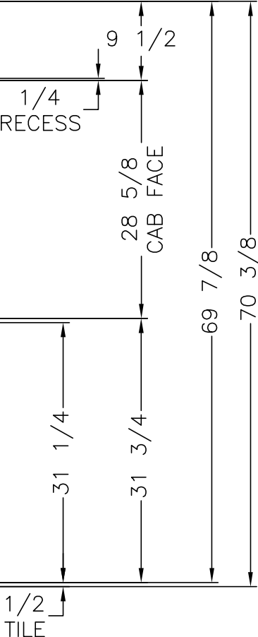
ELEVATION
