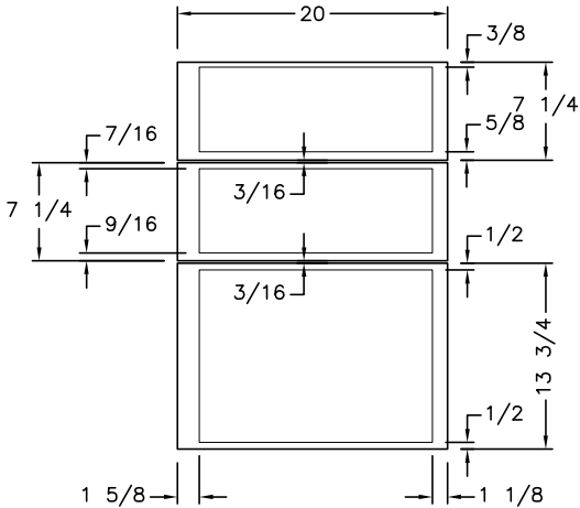
DOOR OVERHANGS
