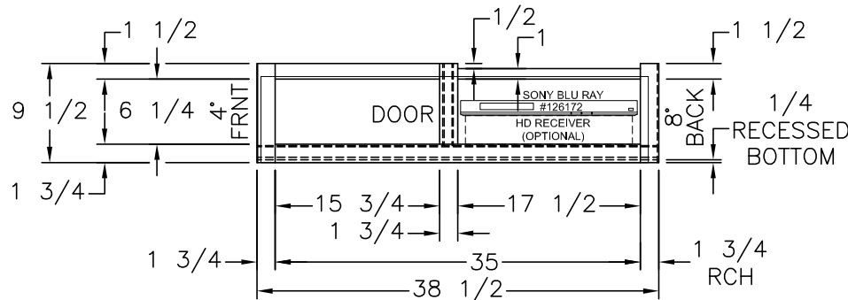
(1) 37 1/8x8 1/4 DOOR (TOP HINGE)
