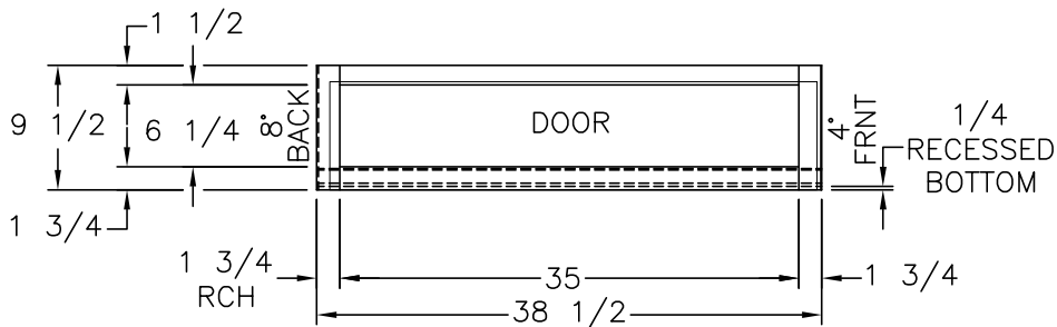
(1) 37 1/8x8 1/4 DOOR (TOP HINGE)
