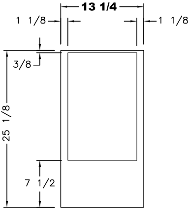
DOOR OVERHANGS
