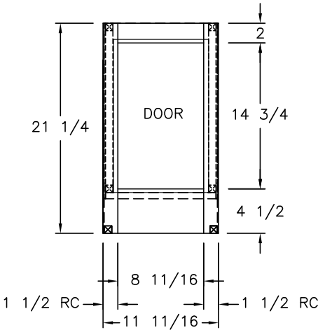
(1) 15 1/2x9 5/8 DOOR
