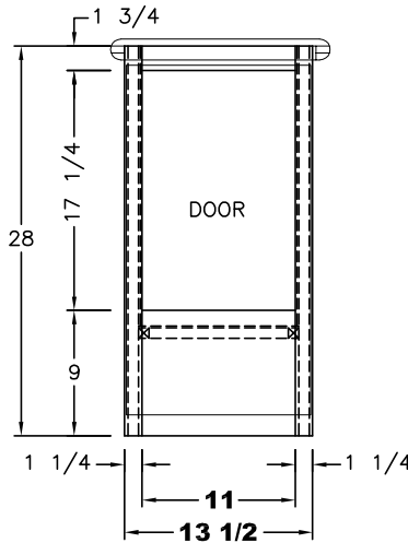
(1) 13 1/4x25 1/8 DOOR
