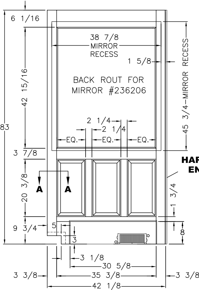
VIEW (D)
