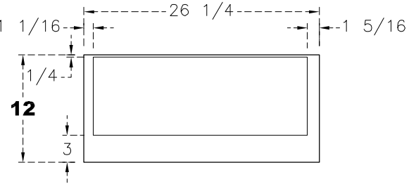
(1) 26 1/4x12 DOOR
