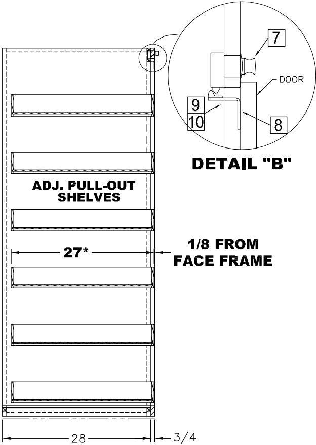
A-A
