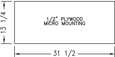
DETAIL 'G'
