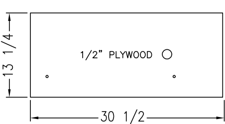
DETAIL 'G'
