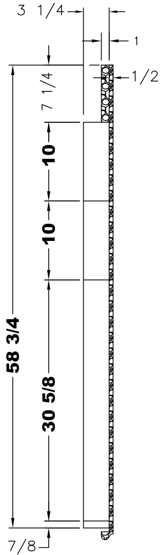
SECTION A-A
