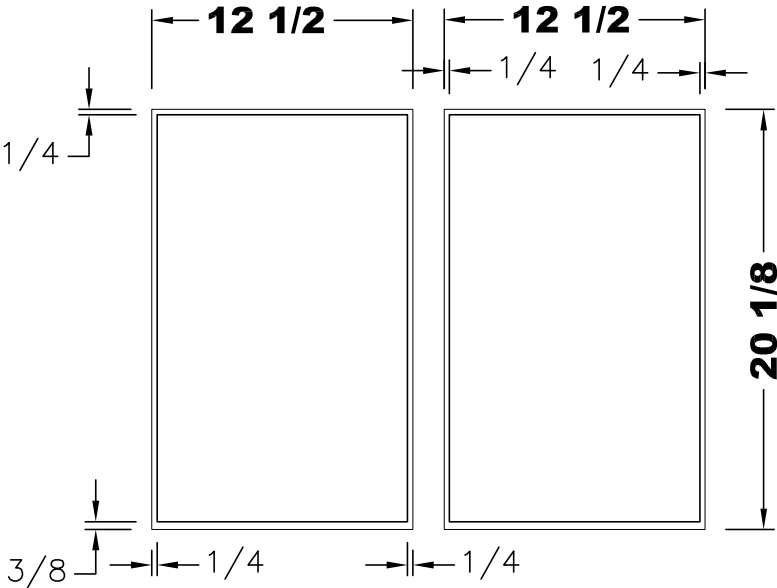
DOOR OVERHANGS
