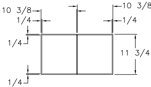
DOOR OVERLAY
