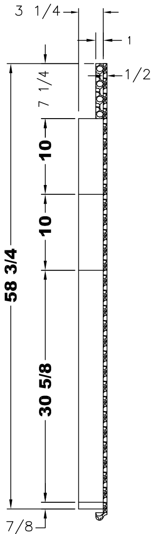
SECTION A-A
