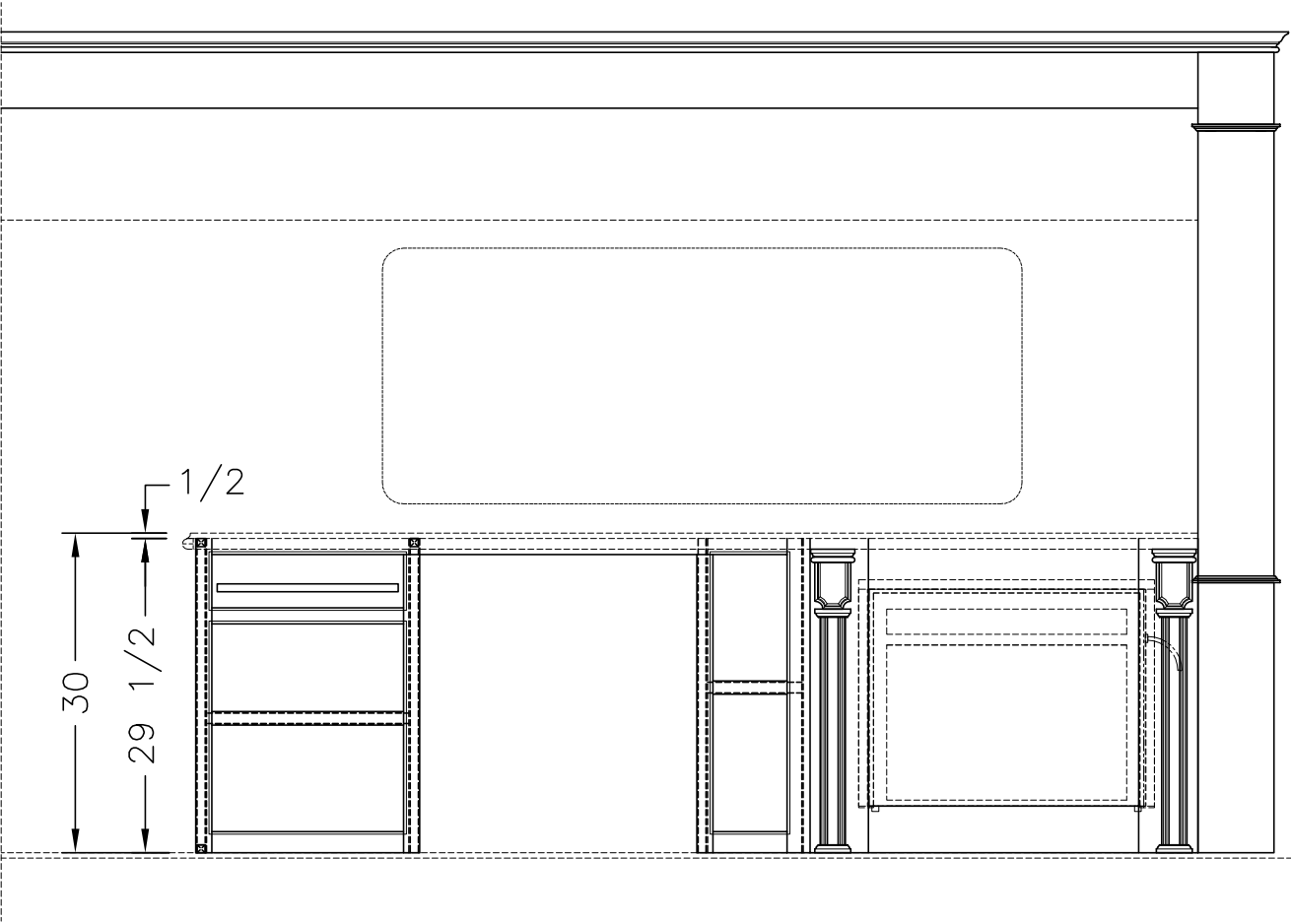
ELEVATION
