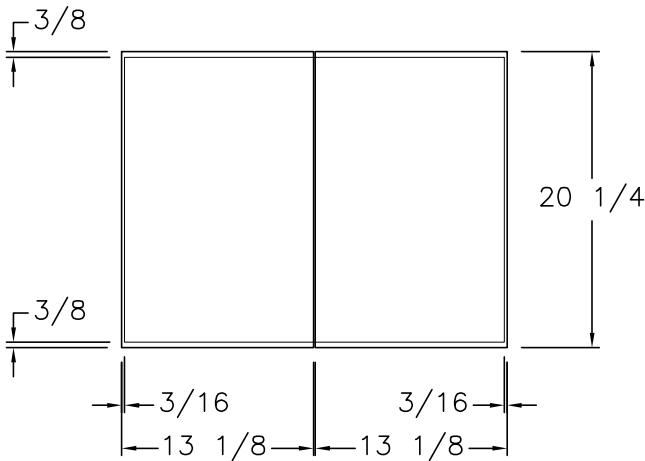
(2) 13 1/4 x 20 1/4 DOORS
