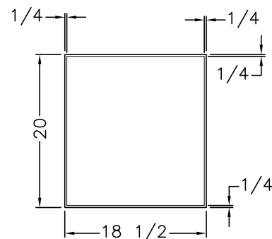
DOOR OVERLAYS
