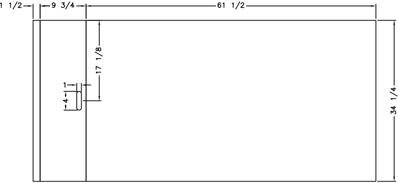
BOTTOM BUNK CNC TOP
