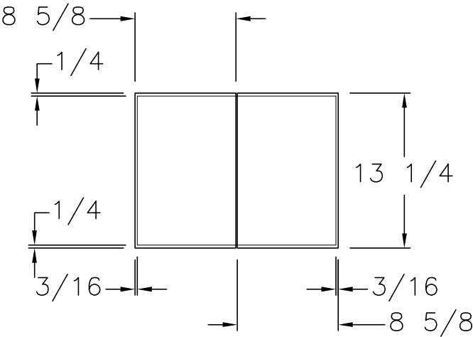
DOOR OVERLAY (B)
