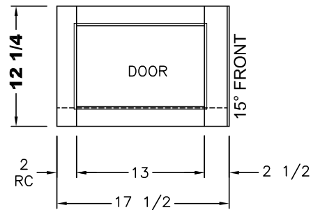
(1) 13 1/2x9 GLASS DOOR TOP HINGE
