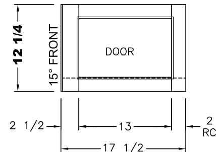
(1) 13 1/2x9 GLASS DOOR TOP HINGE
