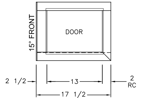
(1) 13 1/2 X 10 3/4 DOOR (TOP HINGE)
