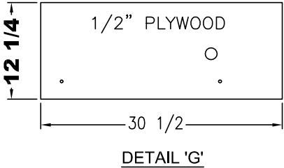
DETAIL 'G'
