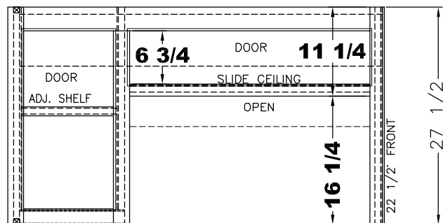
(1) 7 1/4x30 3/4 HINGE DOOR (1) 11 7/8x23 DOOR
