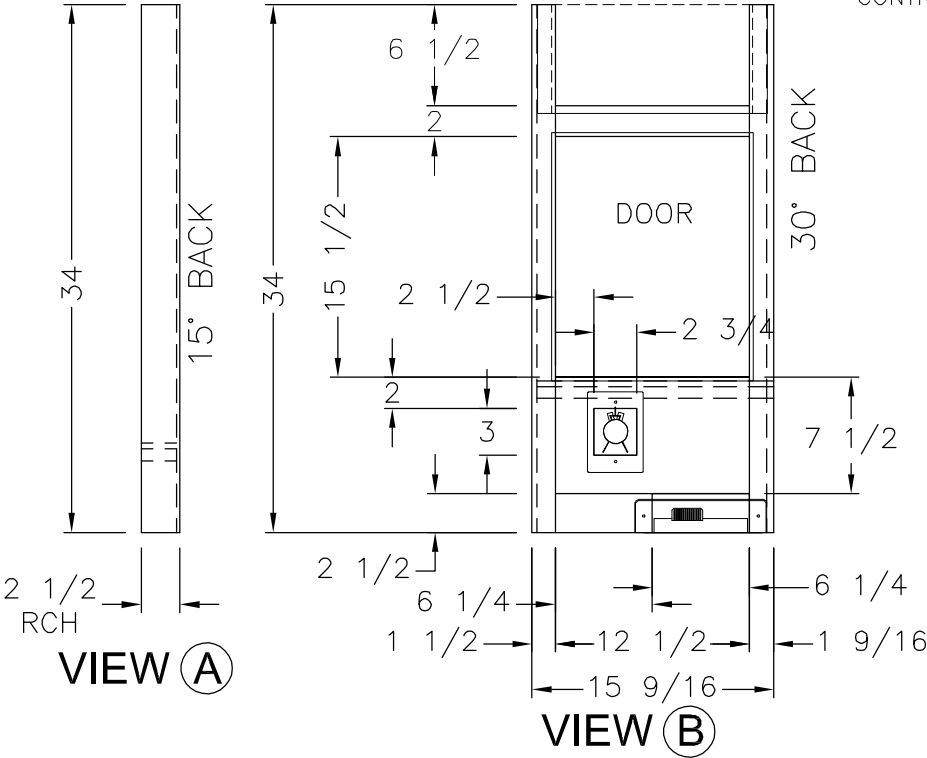
(1) 13x16 DOOR (LFT HG)
