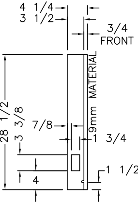
LEG-B (1-REQ'D)
