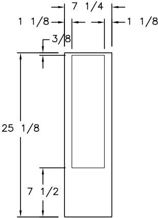
DOOR OVERHANGS
