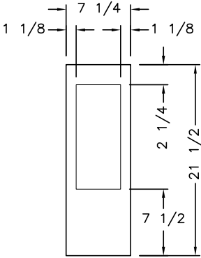
DOOR OVERHANGS
