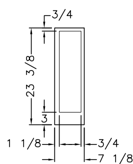
VIEW (D)
