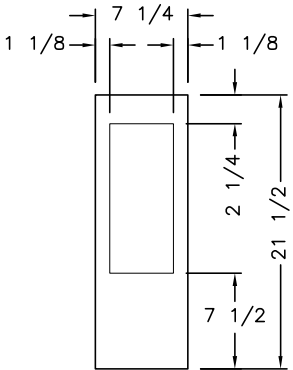
DOOR OVERHANGS
