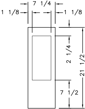
DOOR OVERHANGS
