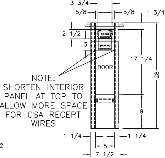
(1) 7 1/4x21 1/2 DOOR
