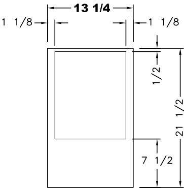
DOOR OVERHANGS
