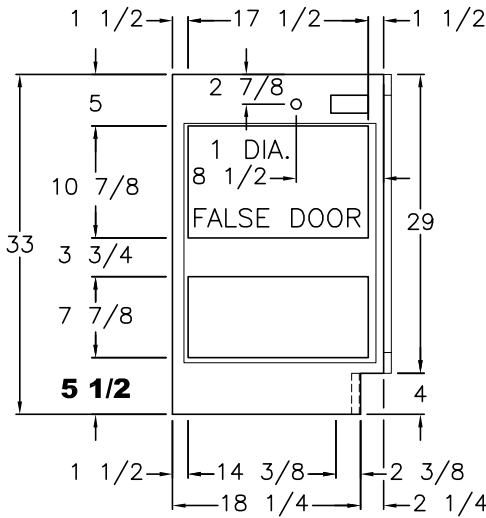
RETURN PANEL (1) 18 5/8x23 1/4 FALSE DOOR
