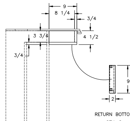
DOOR OVERHANGS
