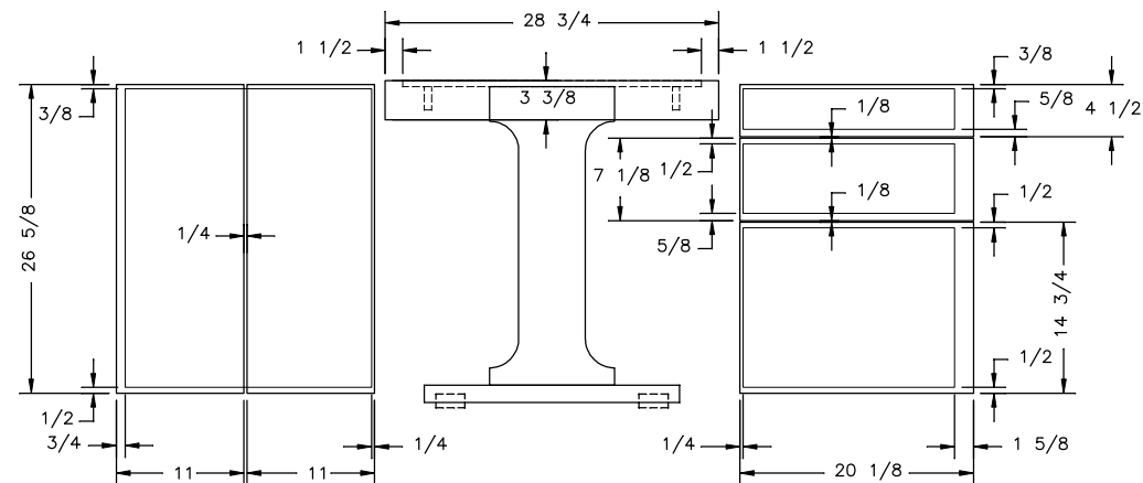
DOOR OVERHANGS
