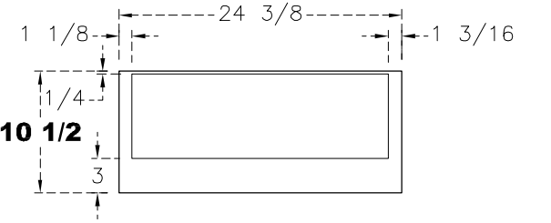
(1) 24 3/8x10 1/2 DOOR
