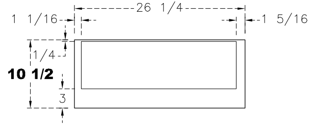
(1) 26 1/4x10 1/2 DOOR
