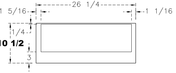
(1) 26 1/4x10 1/2 DOOR
