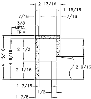
E-E
