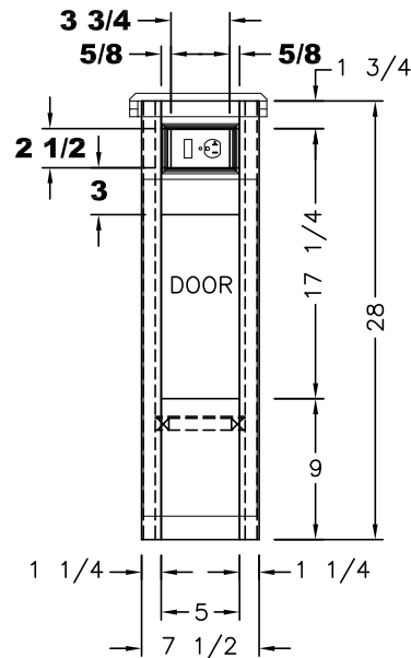
(1) 7 1/4x21 1/2 DOOR
