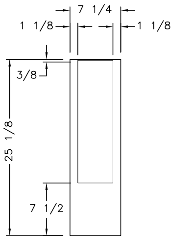
DOOR OVERHANGS
