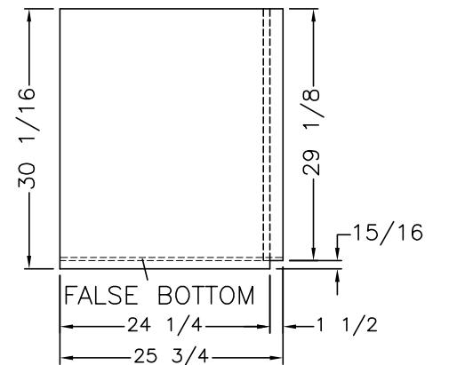
25 3/4 W./ OPT (J560) PARTITION - C
