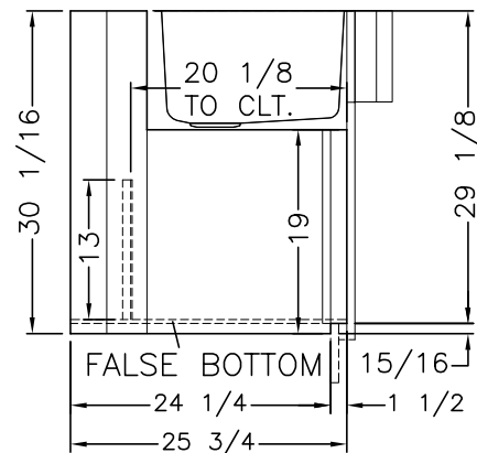
25 3/4 W./ OPT (J560) PARTITION - A
