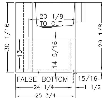
25 3/4 W./ OPT (J560) PARTITION - B
