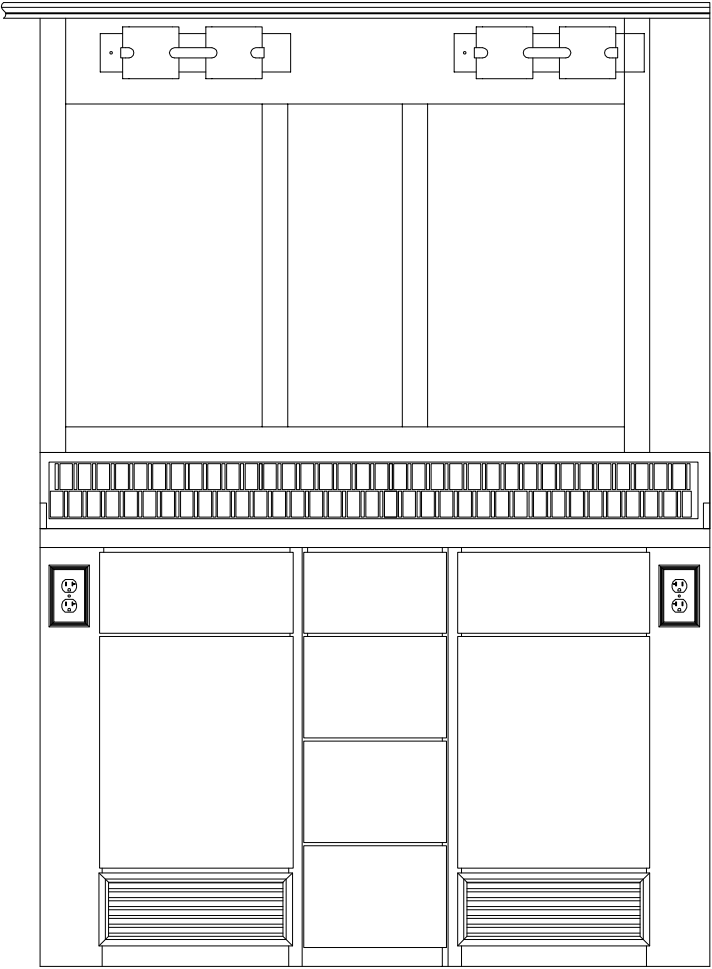
ELEVATION
