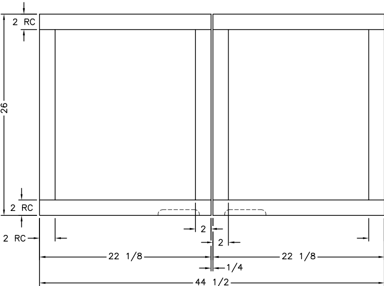
DOOR FRAME
